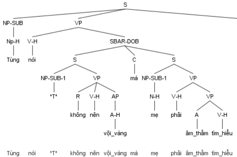
Figure 1. A tree in the Vietnamese Treebank “ Tùng nói *T* không nên vội_vàng mà mẹ phải âm_thầm tìm_hiểu . ” ( Tung suggests that *T* should not be hastily but mother must be silent to find out . )
